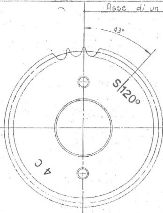
Corona comando albero a cammes di scarico (stampigliata) 41 211 114
