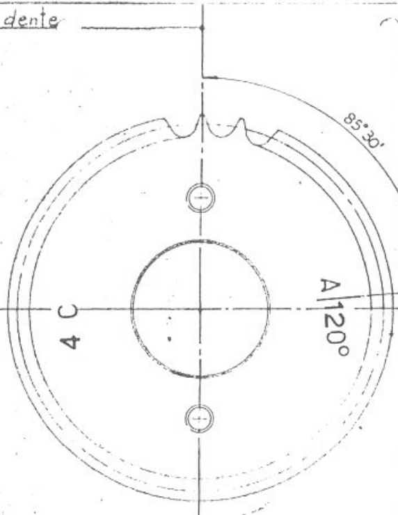
Corona comando albero a cammes di aspirazione (stampigliata) 41 211 115
